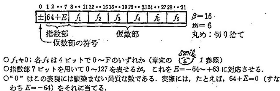
図 1-1 数の内部表現の概念図 (IBM 方式)
